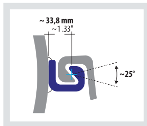
L8n / E22 Larssen / Z
