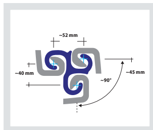
LTn (VTS) Larssen / Z
