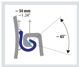
LV22 Larssen / Z
