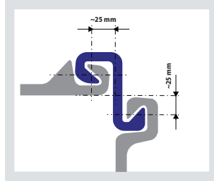
E-20 Larssen / Z
